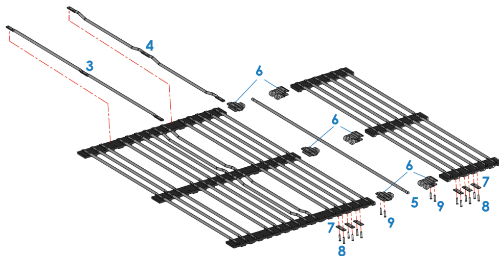
Tweede zeefband
